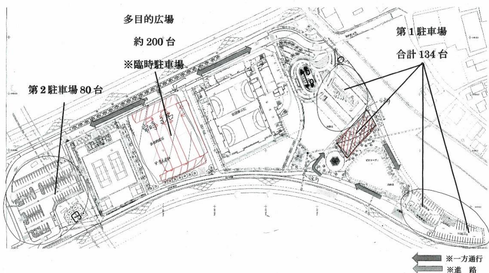
体育館周辺駐車場平面図
